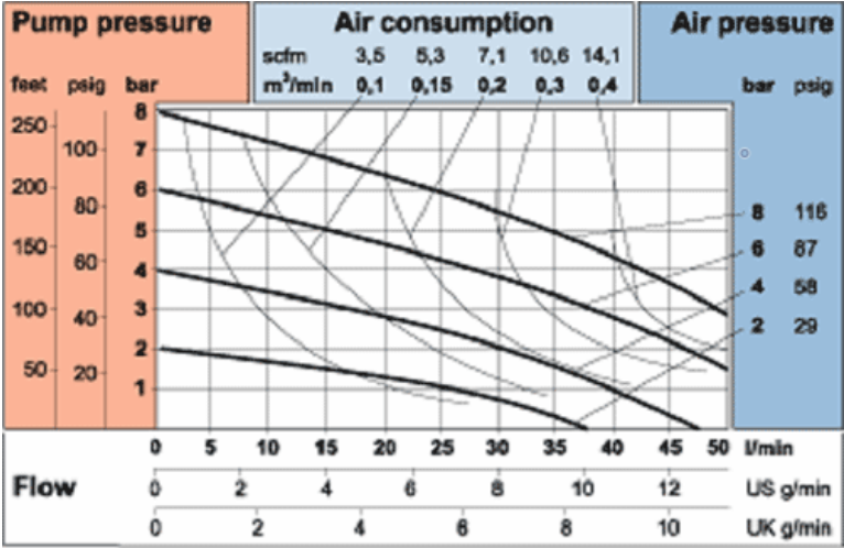
T50 - 50l/min, 1/2"
