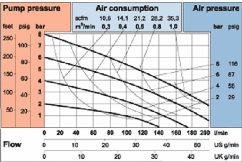
T200 - 200l/min, 1 1/2"
